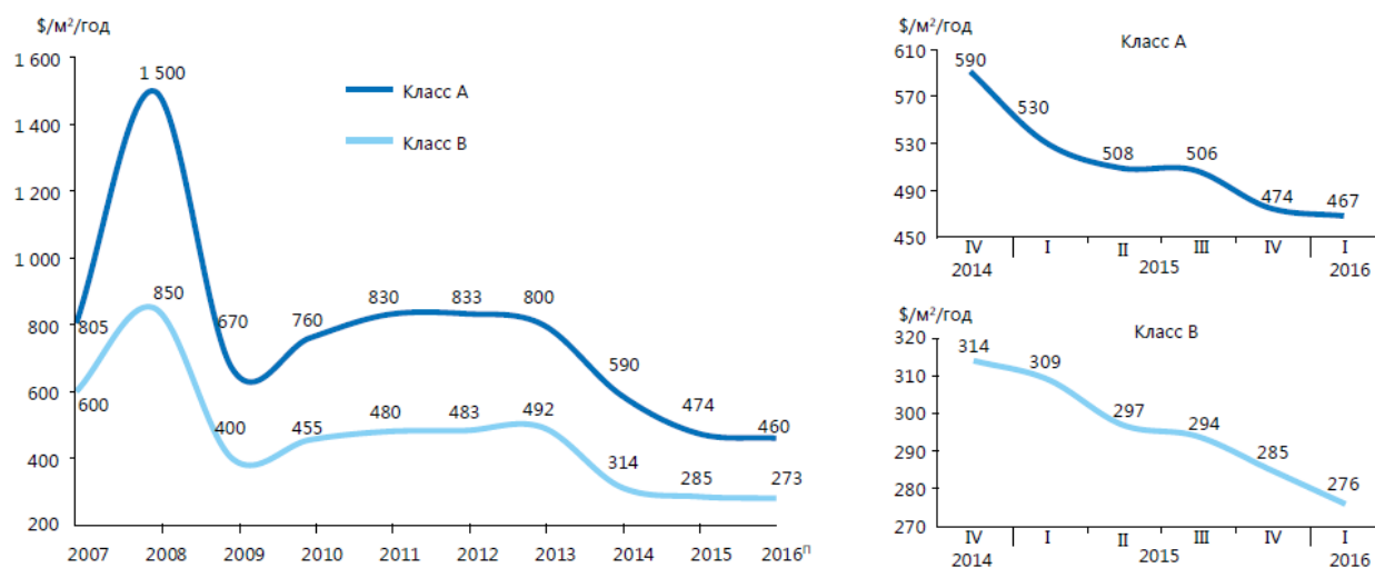
Динамика средневзвешенных запрашиваемых ставок аренды на офисы классов А и В, номинированных в долларах США
